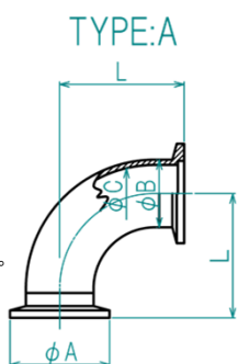
外觀寸法図
