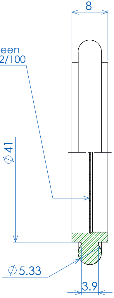
断面図 A-A
