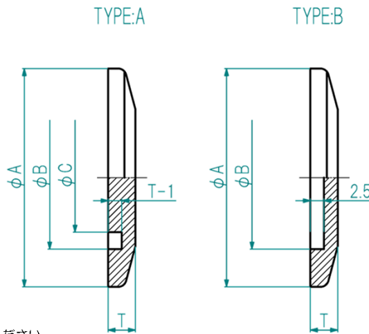
外觀寸法図
