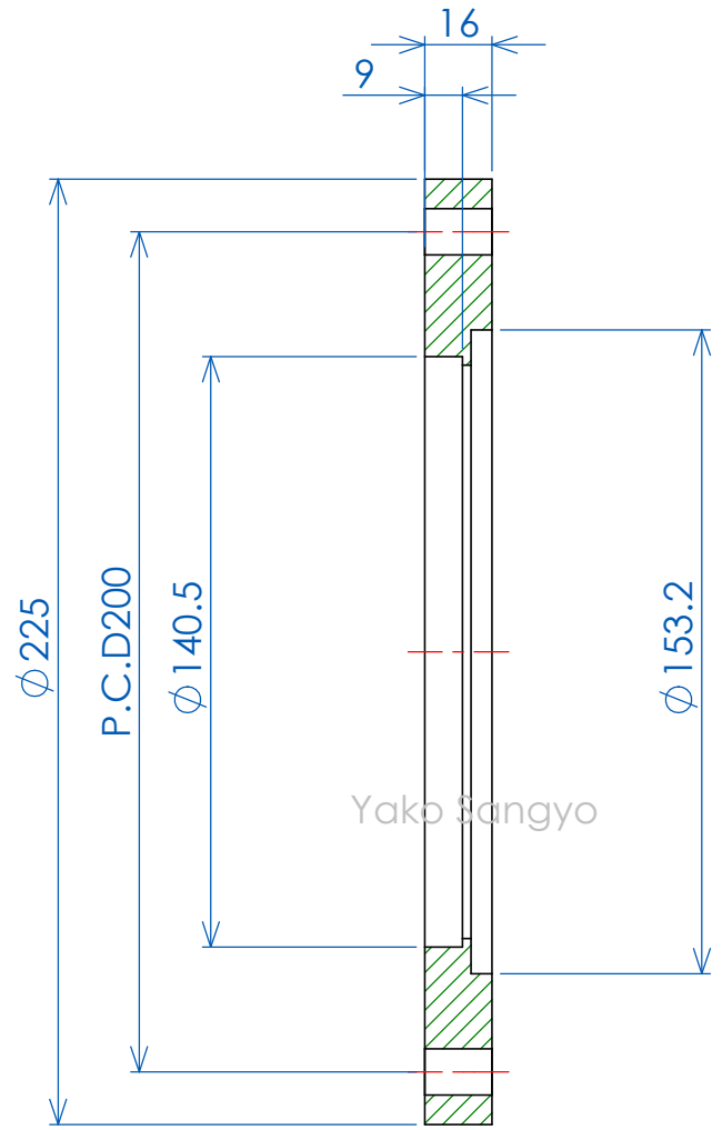
断面図 A-A
