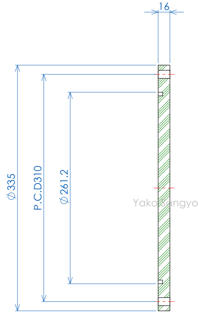
断面図 A-A
