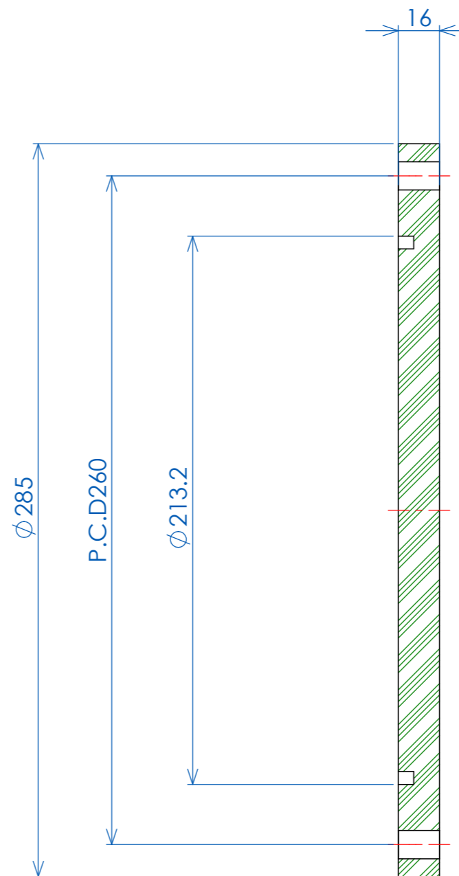
断面図 A-A
