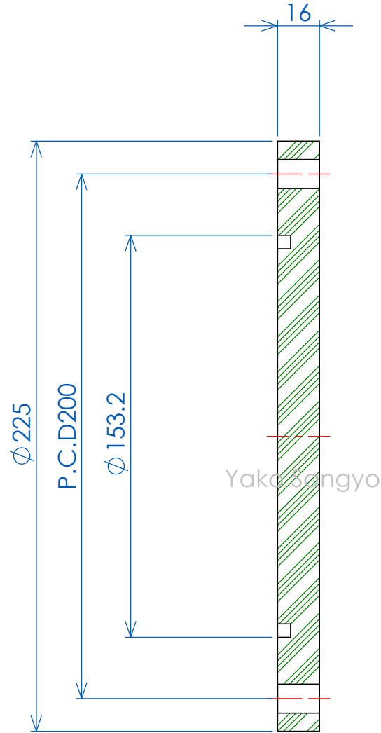
断面図 A-A
