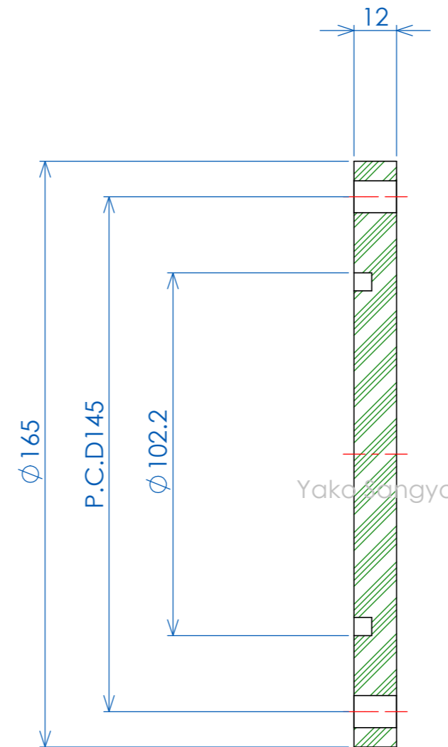
断面図 A-A
