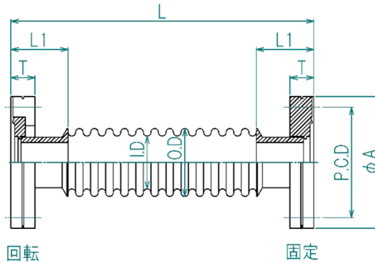
外觀寸法図
