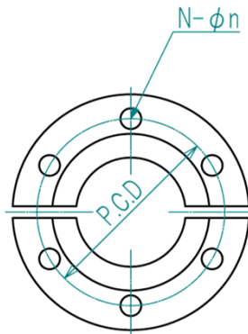
外観寸法図
