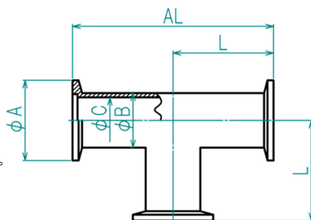
外観寸法図
