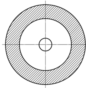
外観寸法図
